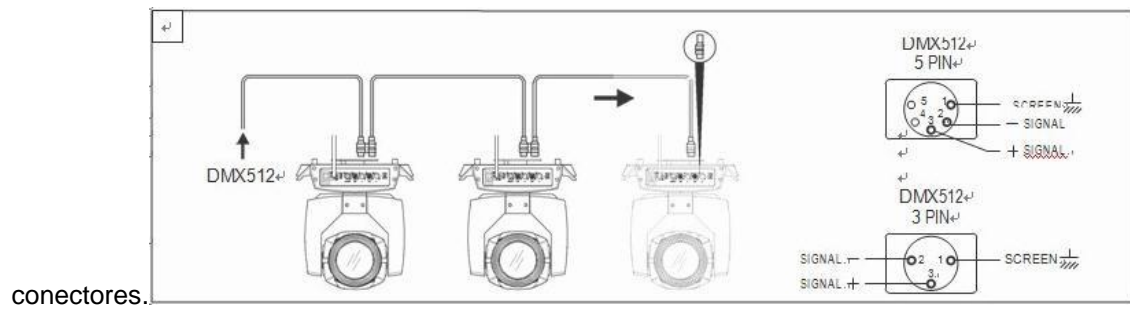
Figura 1 Conexión de cableado de señal DMX
