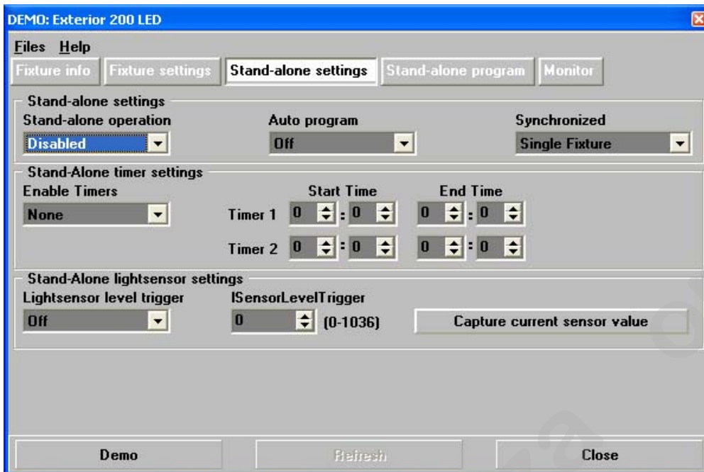
Figura 13: Pantalla de ajustes “Stand- lone”
