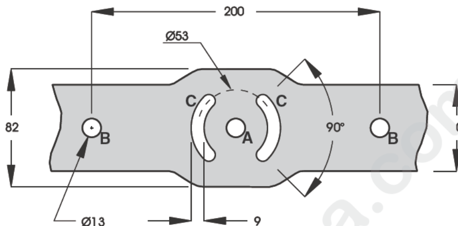
Figura 1: Puntos de fijación del soporte de montaje
