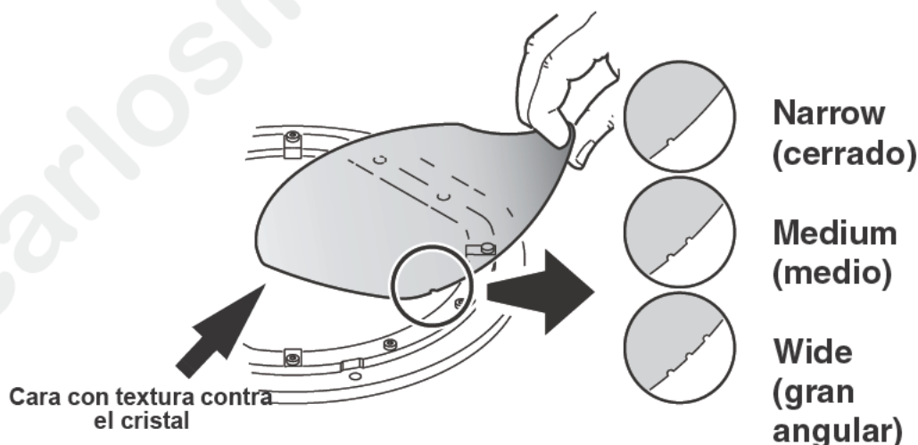
Figura 18: Instalación de un filtro difusor
