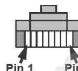
Figura 8 Diagrama de conexión de conector RJ-45
