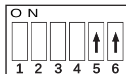
Ajuste de DIP switch para actualización "boot mode"
