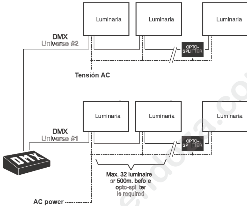
Figura 3: Diagrama esquemático de configuración de cableado
