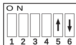
Ajuste normal del DIP switch
