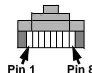
Figura 8: Diagrama de conexión del conector RJ-45
