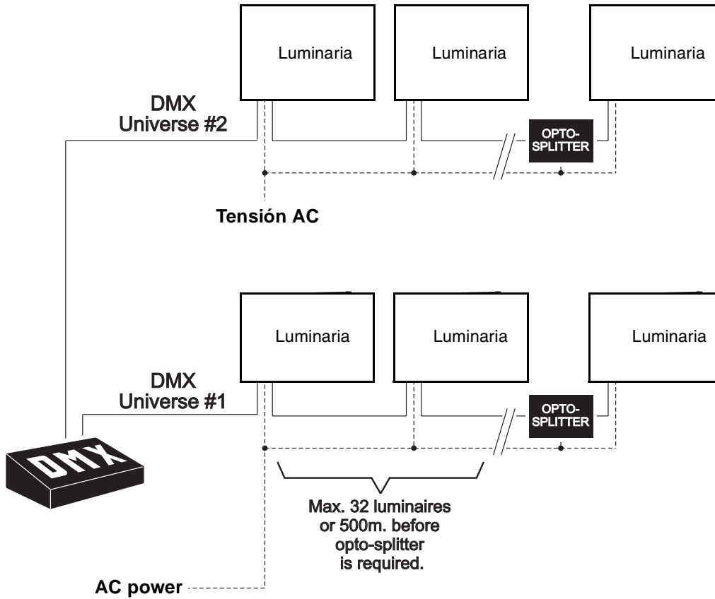
Figura 3: Diagrama esquemático de configuración de cableado
