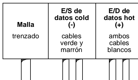
Figura 9: Terminales de datos
