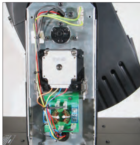
Fig. 19 - Yoke arm
